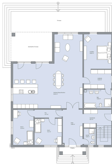
Haus Ortmann Grundriss bemasst EG
