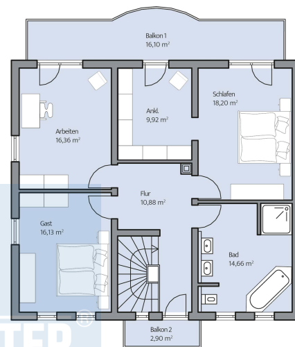
Haus Ernst Grundriss
