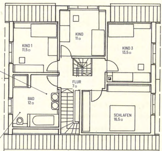
OBERGESCHOSS
