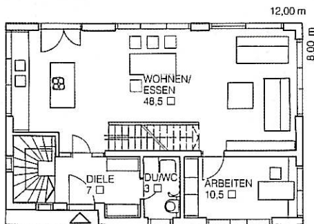
Erdgeschoss
