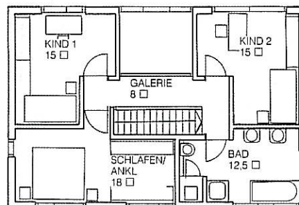
Obergeschoss
